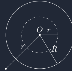
Figura 13.10: La sfera omogenea
