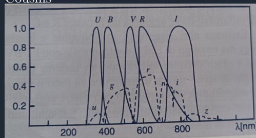
Figura 5.1: Bande del sistema Johnson-Cousins
