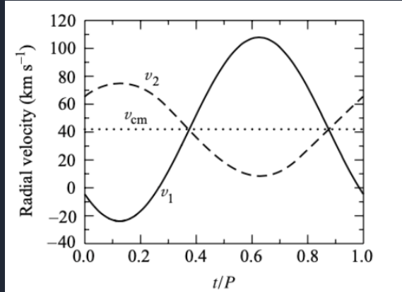
Figura 11.3: Velocità radiale delle stelle binarie
