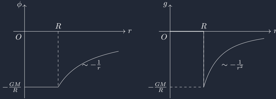
Figura 13.9: Grafici per \phi(r) e g(r) per il guscio sferico
